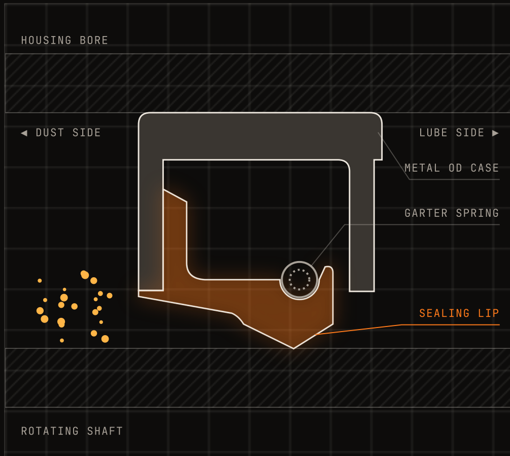
SECTION A-A • METAL OD ROTARY SEAL
